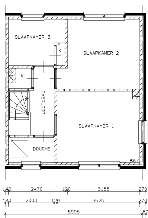
1e VERDIEPING
