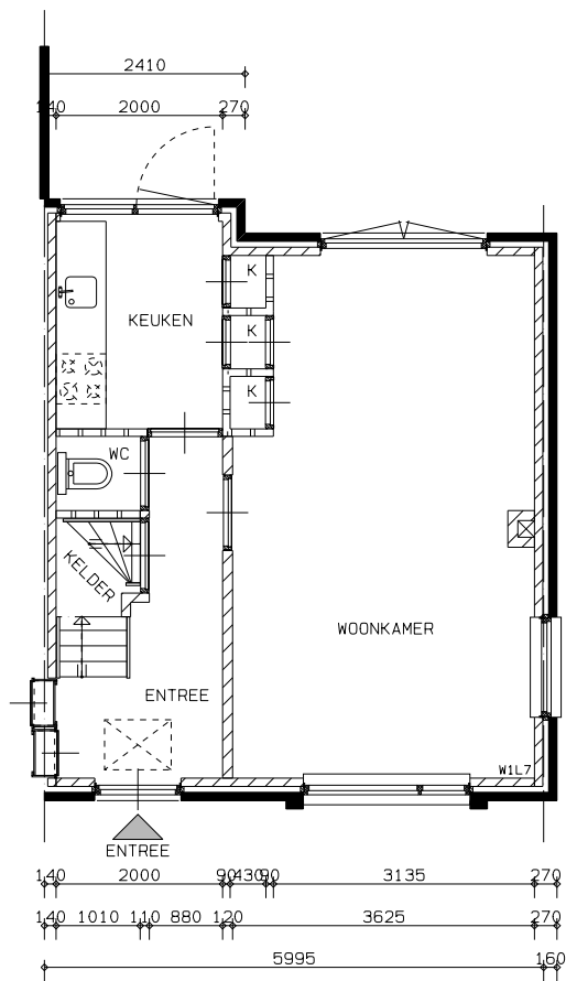
BEGANE GROND
